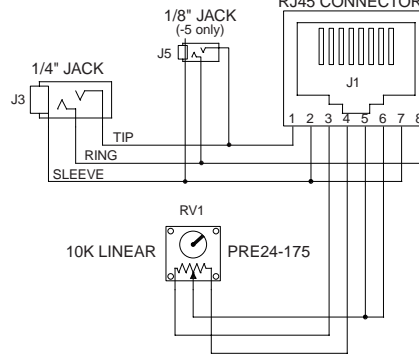
PRE99-1214-3, -4, -5 SCHEMATIC
